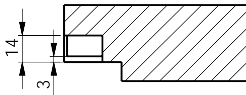
A-A (1 : 2)
